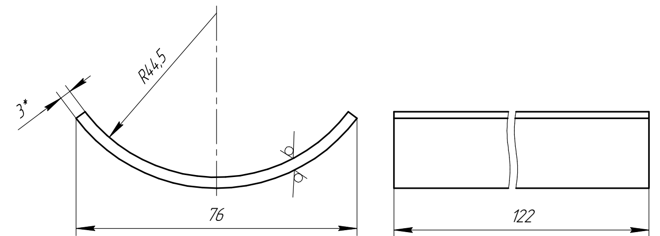
Дет. поз. 3
