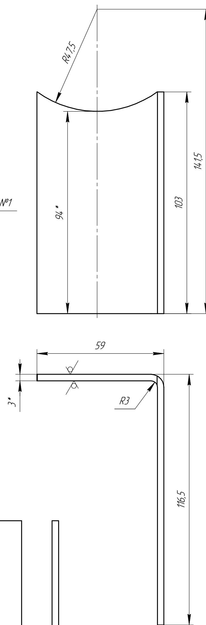
Дет. поз. 2
